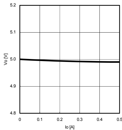
Fig.11 Io-Vo
