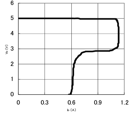
Fig.15 OCP
