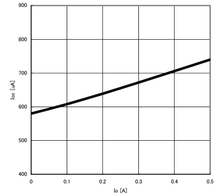
Fig.18 Io-Icc
