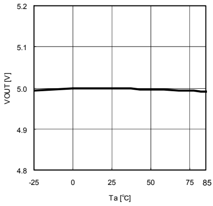
Fig.7 Ta-Vo (Io=0mA)
