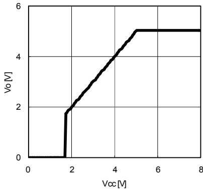
Fig.13 Vcc-Vo (Io=0mA)
